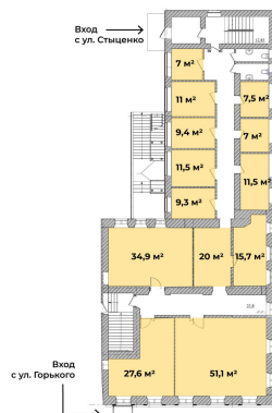
1 этаж
